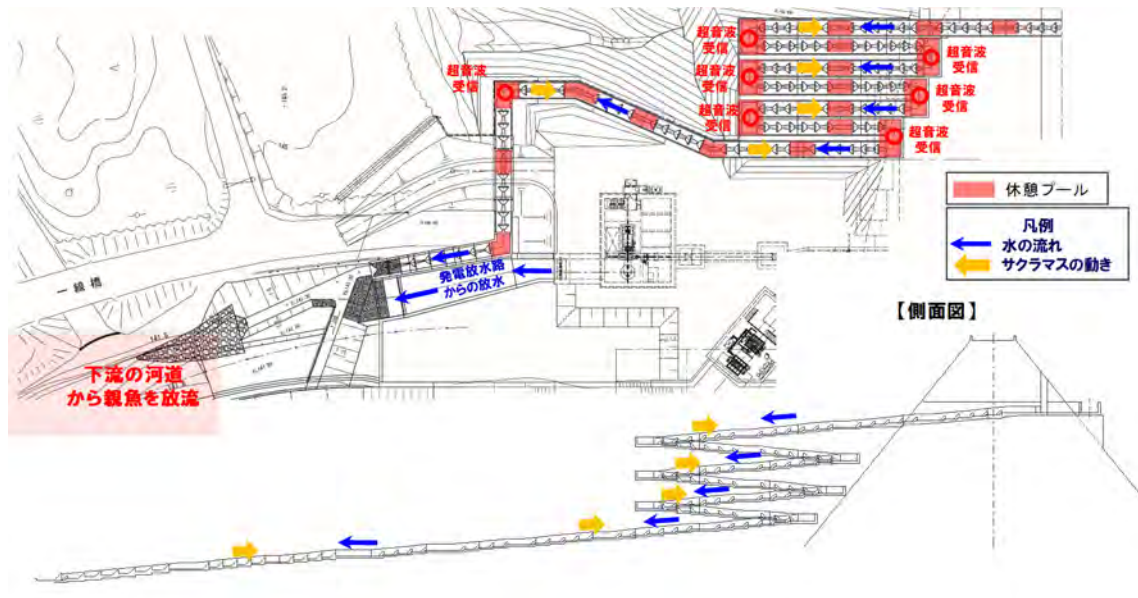
図 - 38 階段式魚道のサクラマス上り調査概要図
