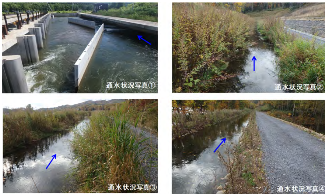
写真- 18 本川との接続箇所を含むバイパス水路全川の流況
