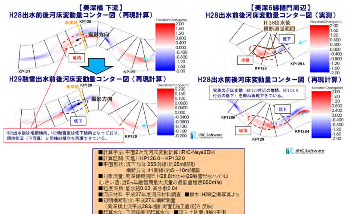
図-57 平面 2 次元河床変動解析による現地状況の再現計算
