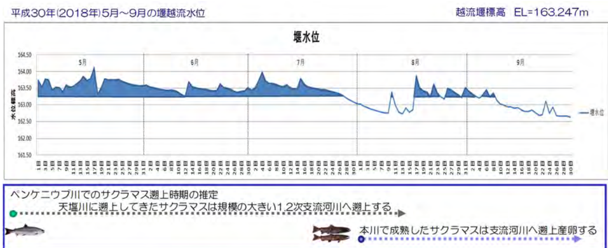
図- 16 ペンケニウプ川取水施設天端高以上の河川水位状況と親魚遡上状況
