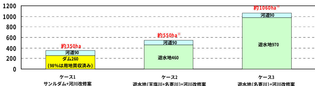
図 6-2-3 用地補償面積の比較
