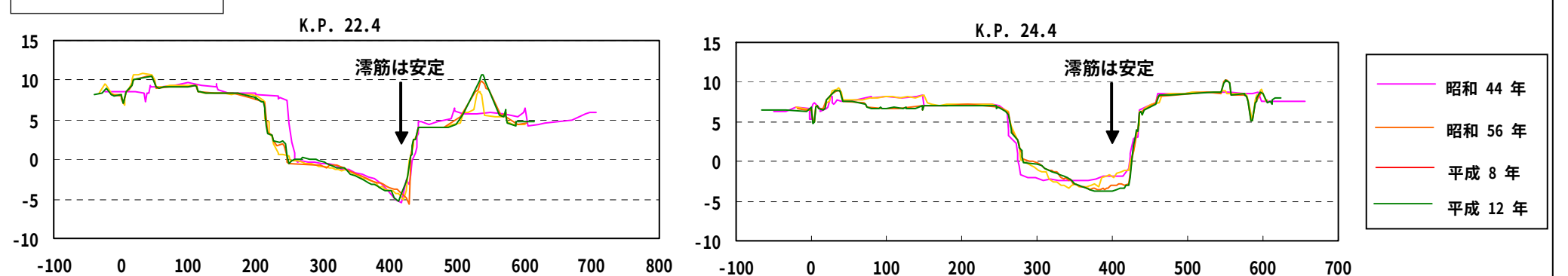
図 2-1-12(3) 河川特性の分析 (天塩川下流域)
