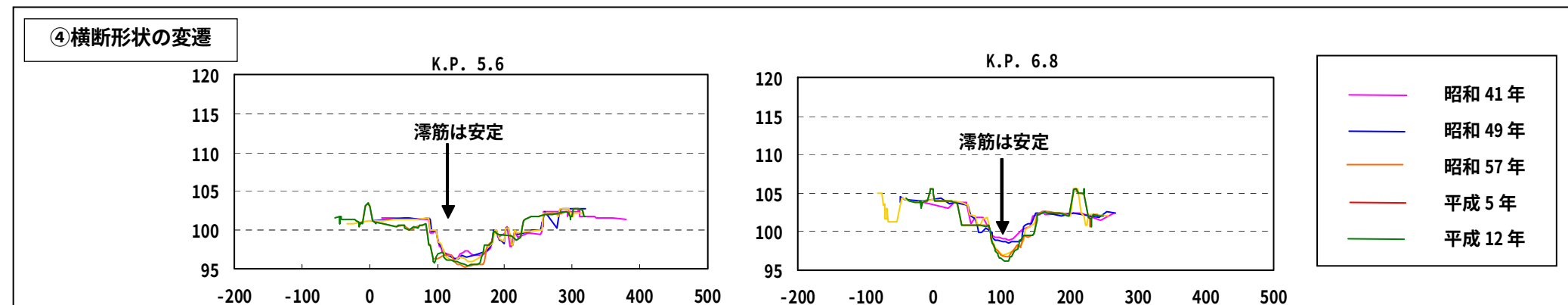
図 2-1-12(4) 河川特性の分析(名寄川)
