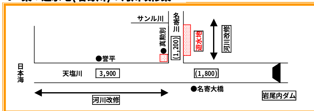
図 5-1-1 治水対策案の比較
