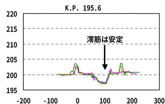
図 2-1-12(1) 河川特性の分析(天塩川上流域)
