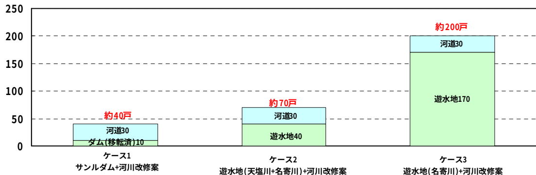
図 6-2-2 移転家屋数の比較
