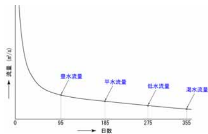
図 4-2-2 天塩川本支川の現在の流況
