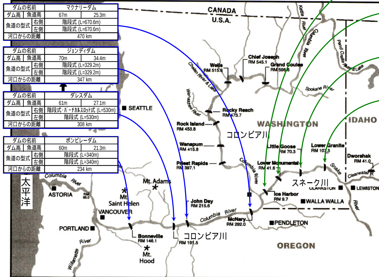
アメリカコロンビア川の ボンビレーダムにおける 階段式魚道
