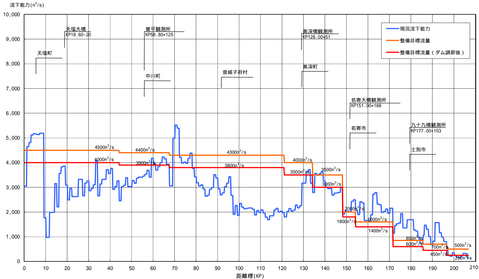
天塩川流下能力図
