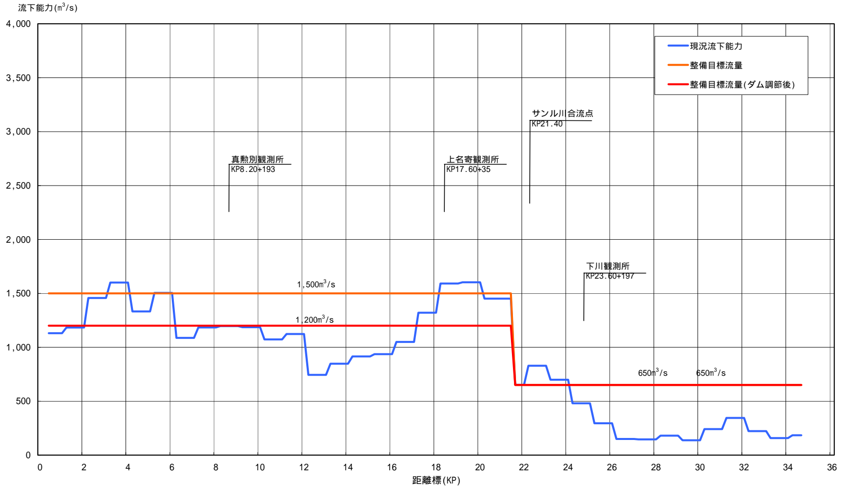
名寄川流下能力図
