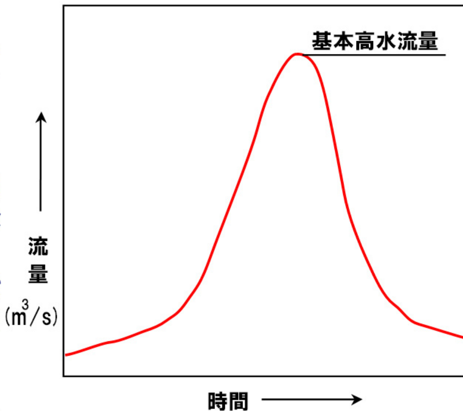
基準地点におけるハイドログラフ
