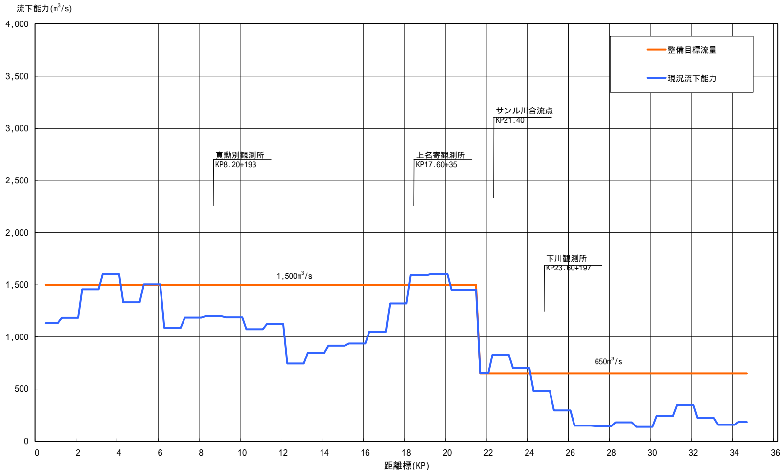
名寄川流下能力図
