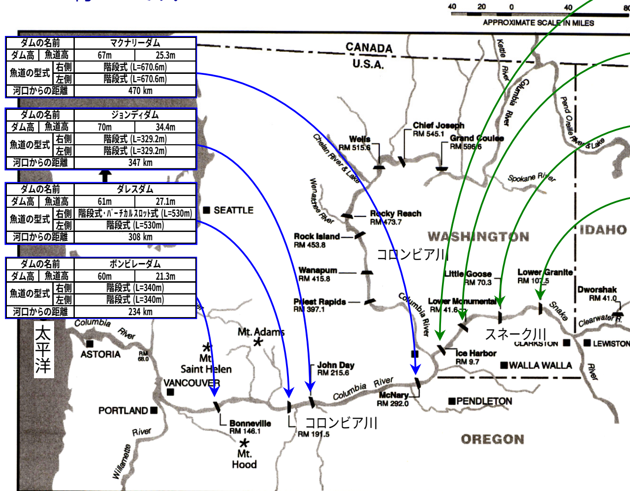
アメリカコロンビア川の ボンビレーダムにおける 階段式魚道
