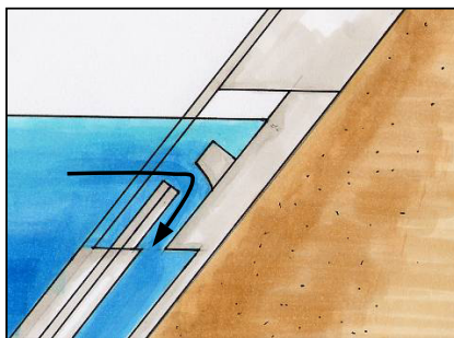
中層から取水
