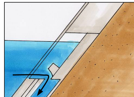
底層から取水
