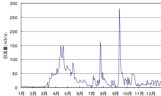
平成13年九十九橋日流量グラフ
