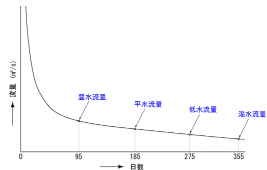
日流量の年間の状況(流況)
