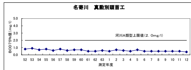
天塩川BOD75%値推移図
