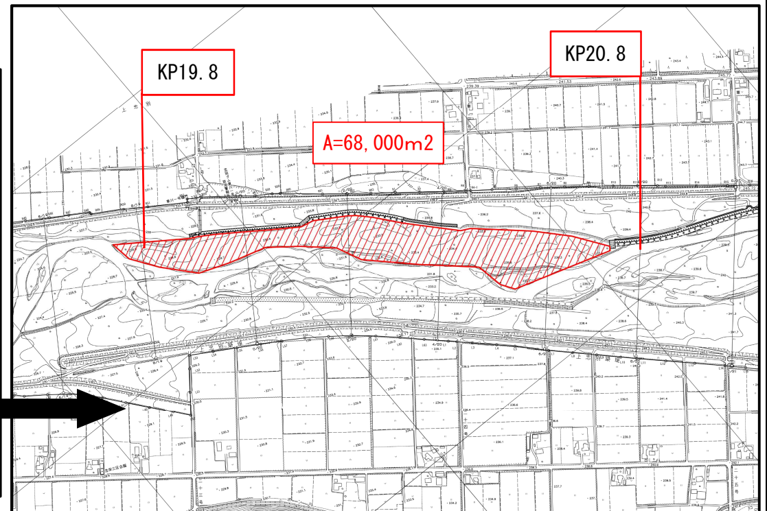
平面図
