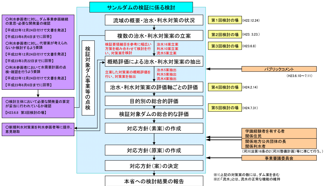
図 1.1.1サンルダム建設事業の検証に係る検討フロー
