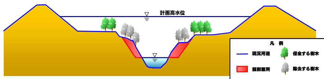
図 4.2.11 河道内の樹木の伐採のイメージ
