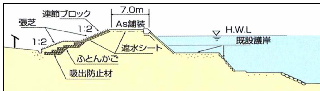
決壊しづらい堤防の例（アーマーレビー工法の概要）
