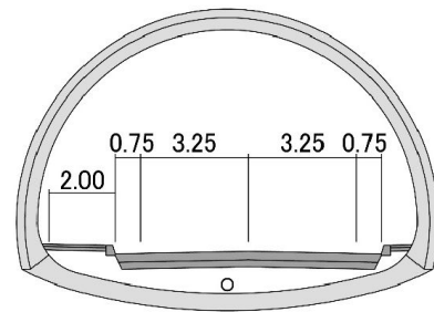
トンネルの道路幅員 (単位:m)
