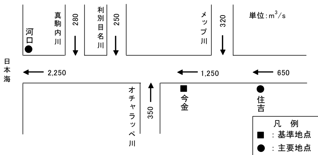
図 1-4 後志利別川水系河川整備基本方針における後志利別川流量配分図
