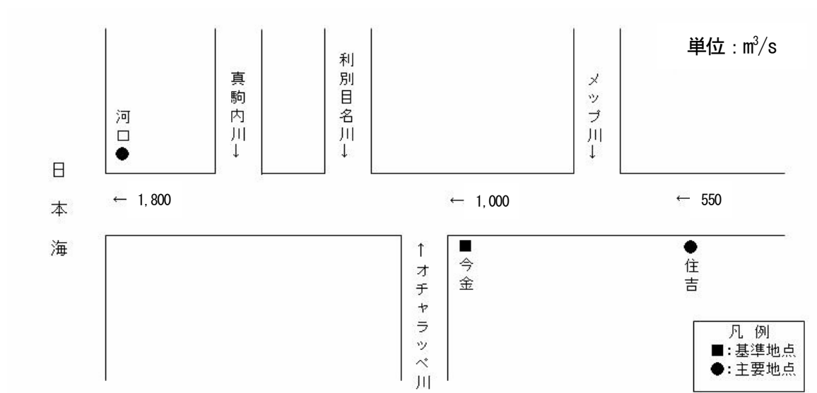
図 1-16 主要な地点における河道への配分流量 (単位 : \text{m}^3/\text{s} )
