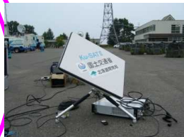
衛星小型画像伝送装置
