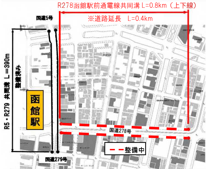
R278 函館駅前通電線共同溝整備イメージ
