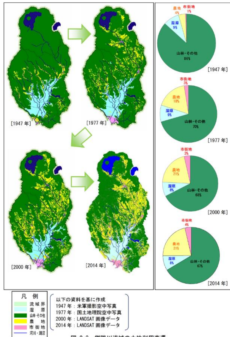
図 2-2 釧路川流域の土地利用変遷
