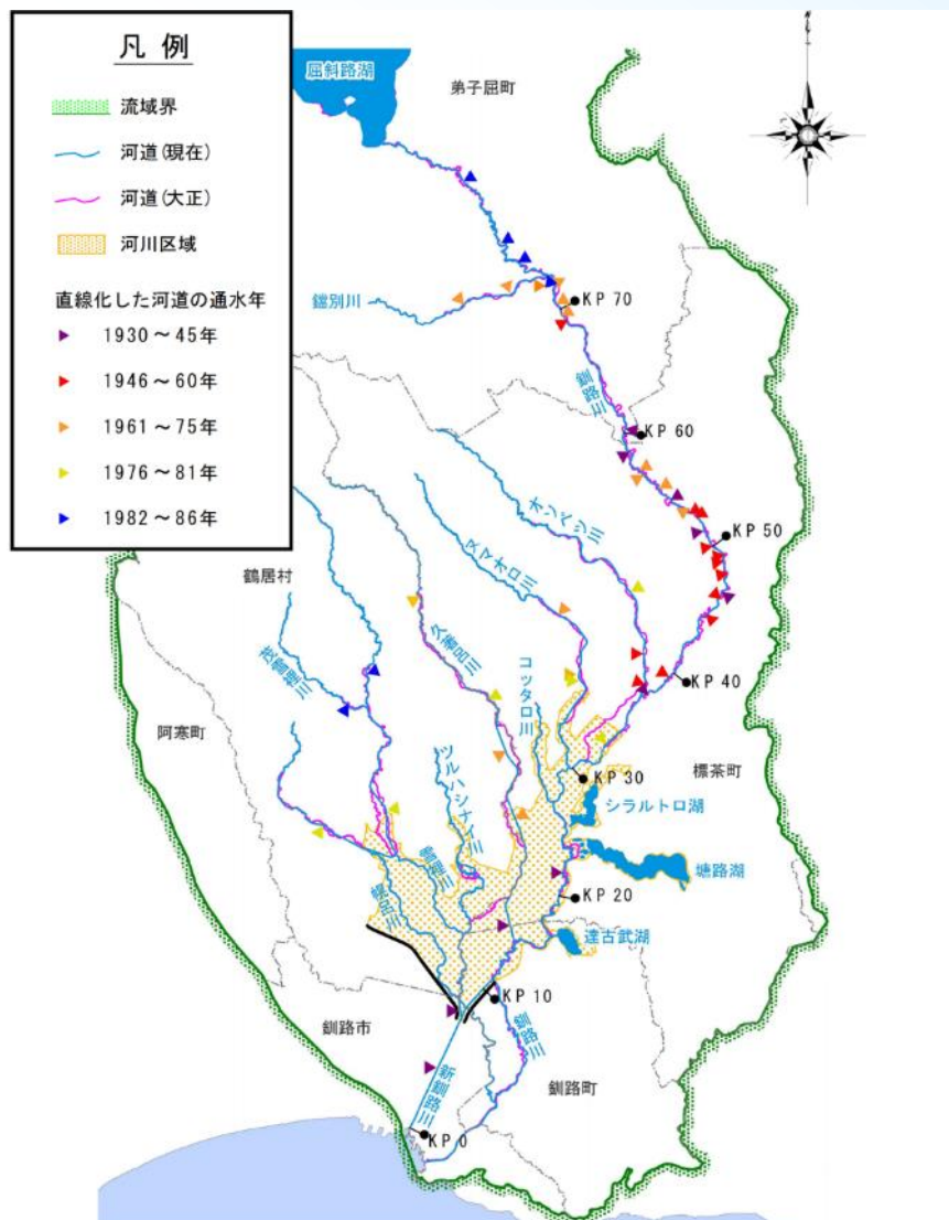
図 2-1 釧路川流域河道変遷図(大正と現在の比較)
