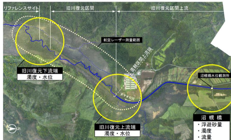
図 3-24 土砂流出量調査箇所位置図
