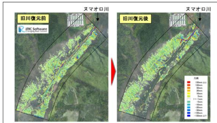
図 3-14 氾濫解析による堆積厚分布図の例 (既往最大規模程度の実績洪水(ピーク流量 96m 3 /s)での結果)
