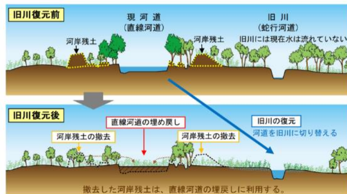
図 3-7 実施手法のイメージ
