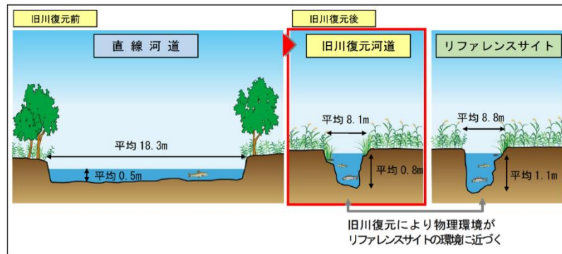
図 3-20 横断形状のイメージ図
