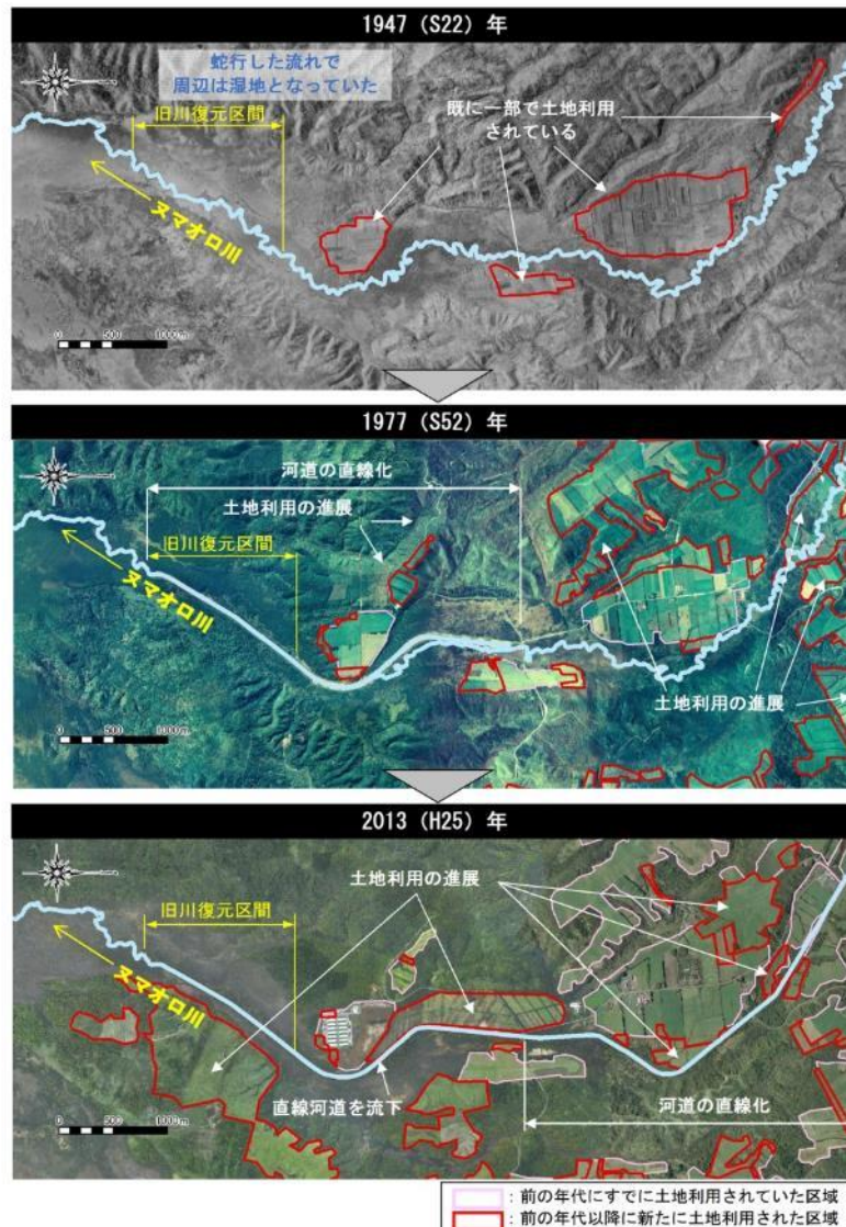
図 3-2 ヌマオロ川と周辺土地利用の変遷
