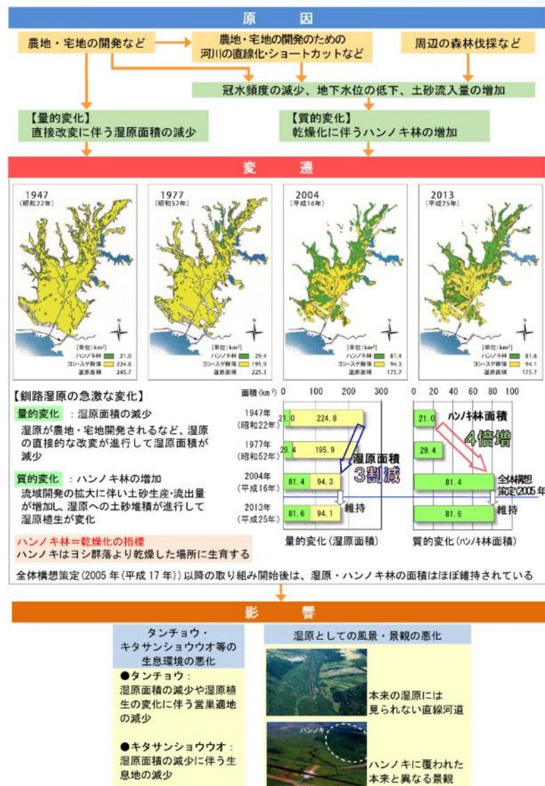
図 2-3 湿原植生の変化の原因と変遷
