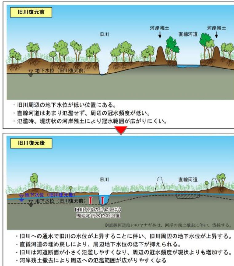
図 3-16 地下水位上昇のイメージ
