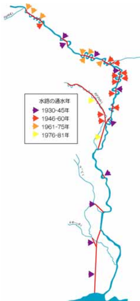
釧路川本川の直線化部分と年代 (釧路開発建設部 2004 を改変)
