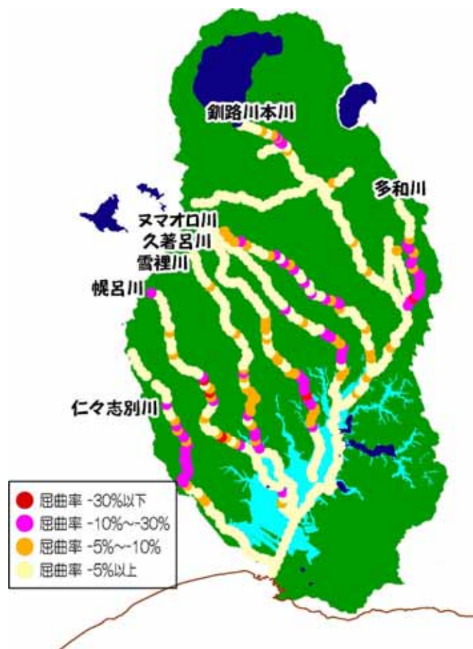
主要な河川における 1950 年から 2000 年の間の 屈曲率の変化 (金子・吉村 2004 を改変)
