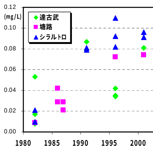
東部3湖沼の水質の経年変化 (全リン量、高村ほか 2003)
