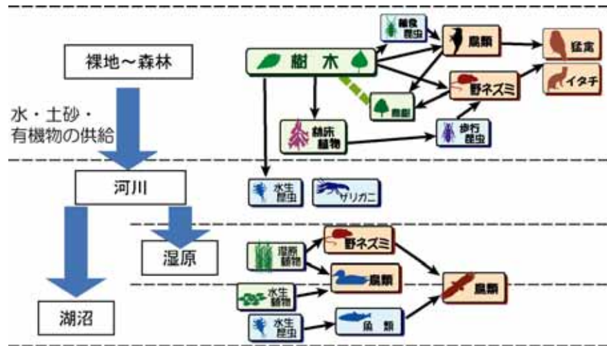
森林生態系とその下流に位置する湿原生態系の構成の例
