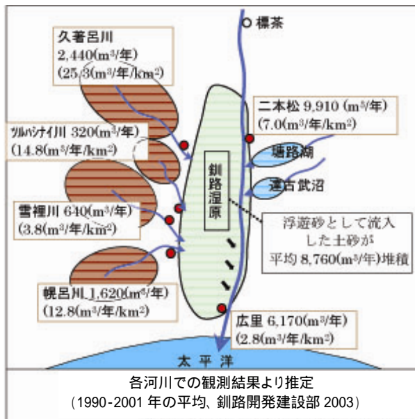
図5-10.主要河川の浮遊砂の収支
