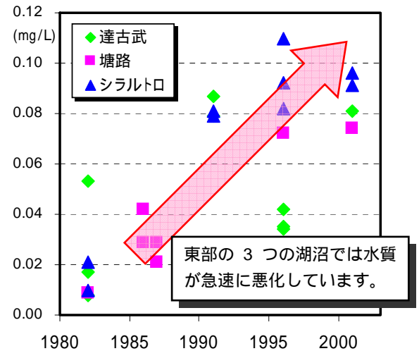
図5-9.東部3湖沼の水質の経年変化 (全リン量、高村ほか 2003)
