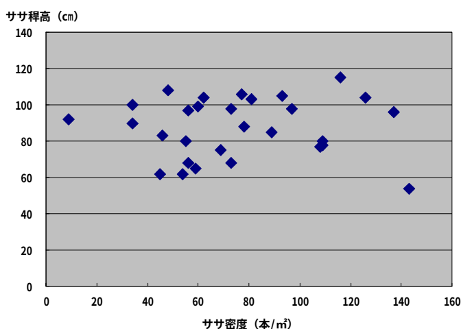
図 3-4-2 ササ密度と稈高の分布
