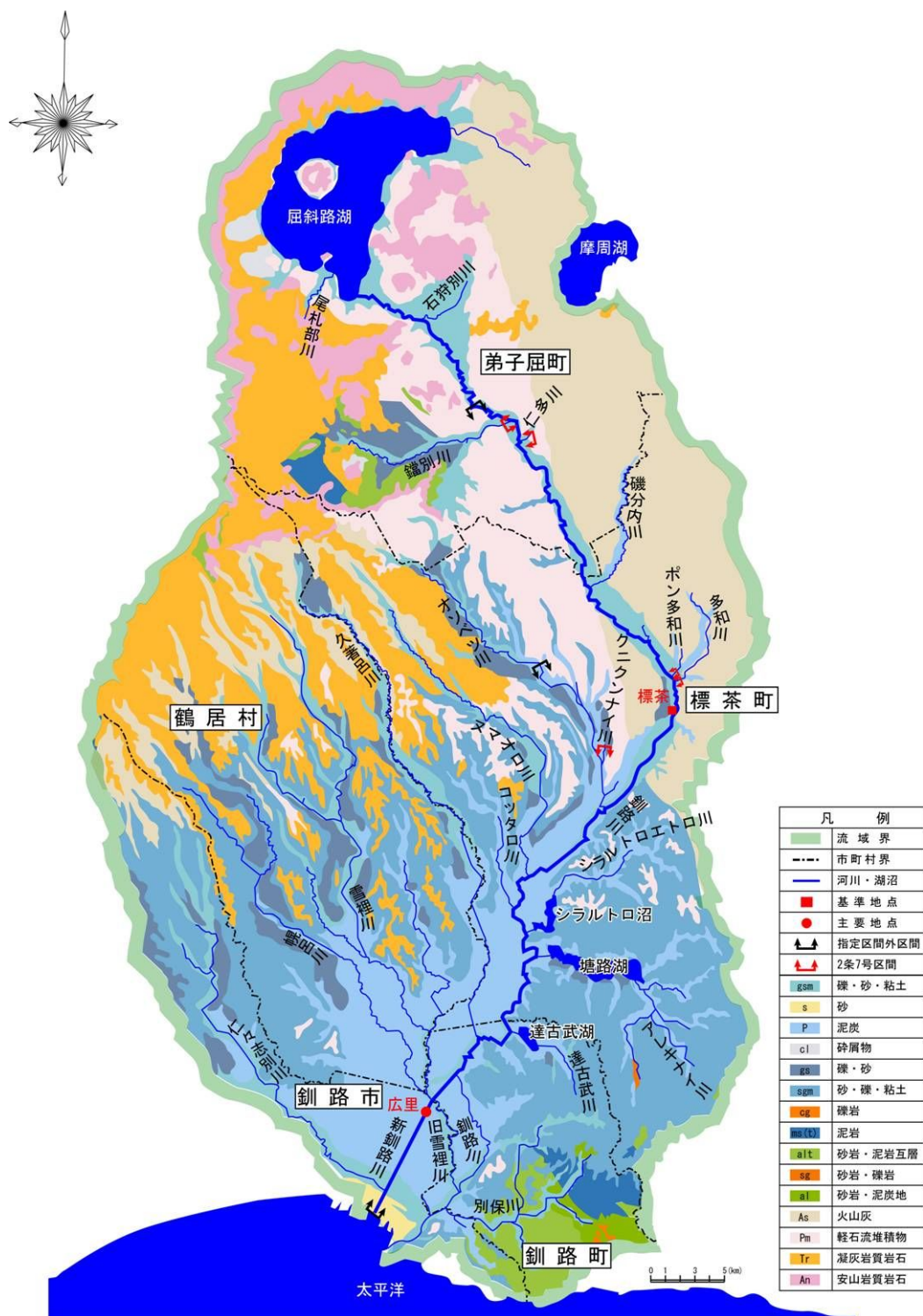
図 1-3 地質図
