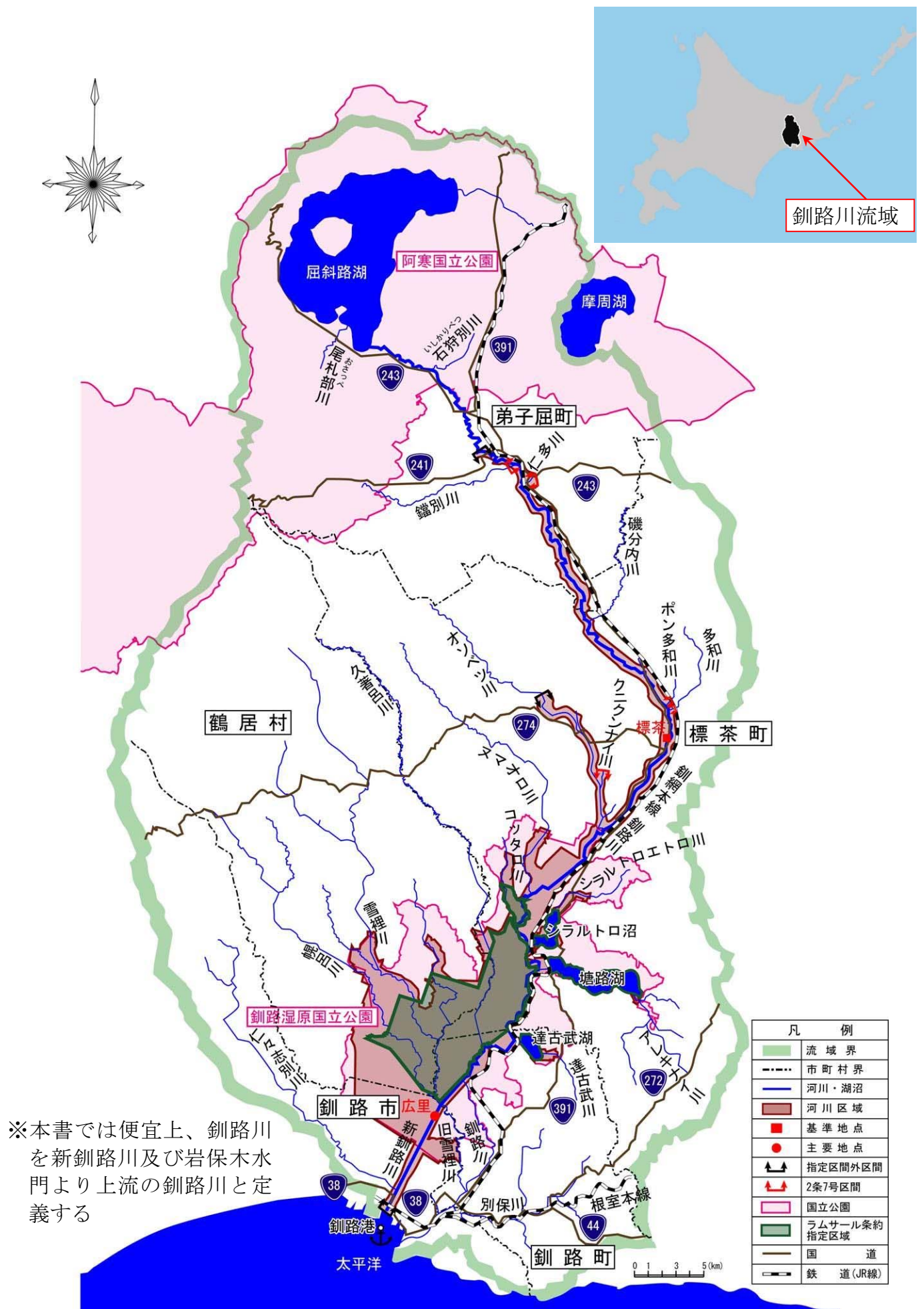
図 1-1 流域図
