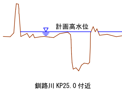
鉏路川計画横断面図 (3/8)
