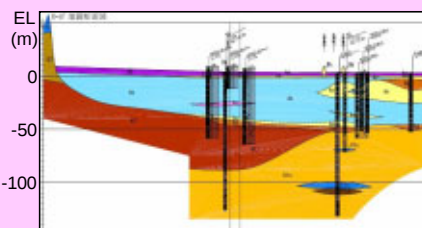
D-D' 断面
