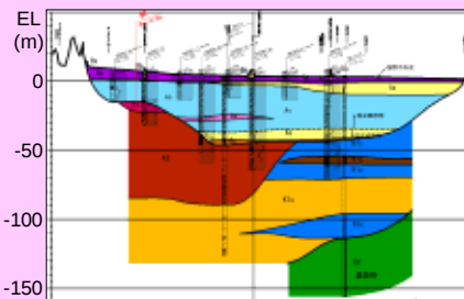
C-C' 断面
