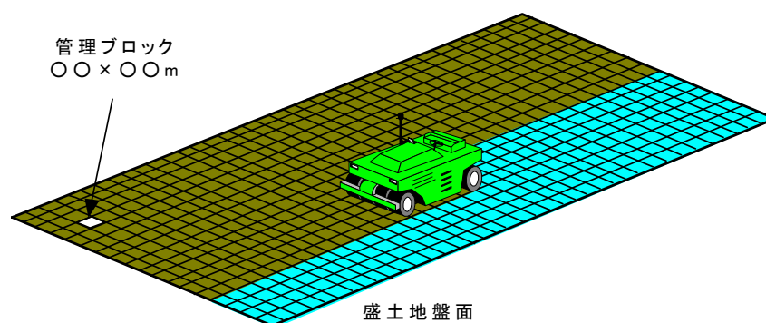
図-1 管理ブロックの概念図
