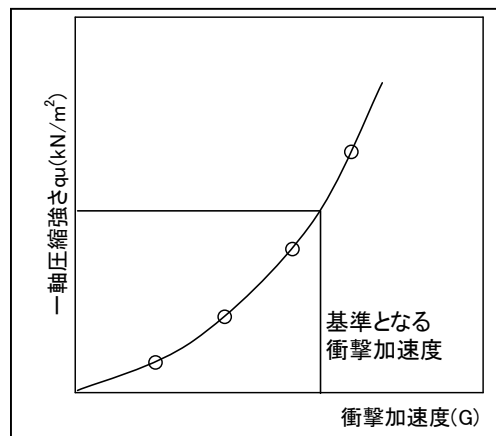
図－4 セメントや石灰などの 固化材により 改良した試料の基準となる衝撃加速度
