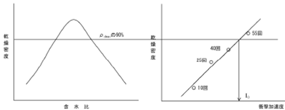
図-2. a 基準となる衝撃加速度
