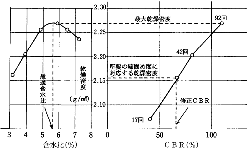
乾燥密度・含水比・CBR関係図
