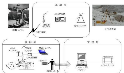
図-3 走行軌跡データの通信経路（GPS の例）
