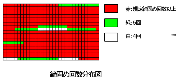
図-5 締固め回数分布図の概念図
