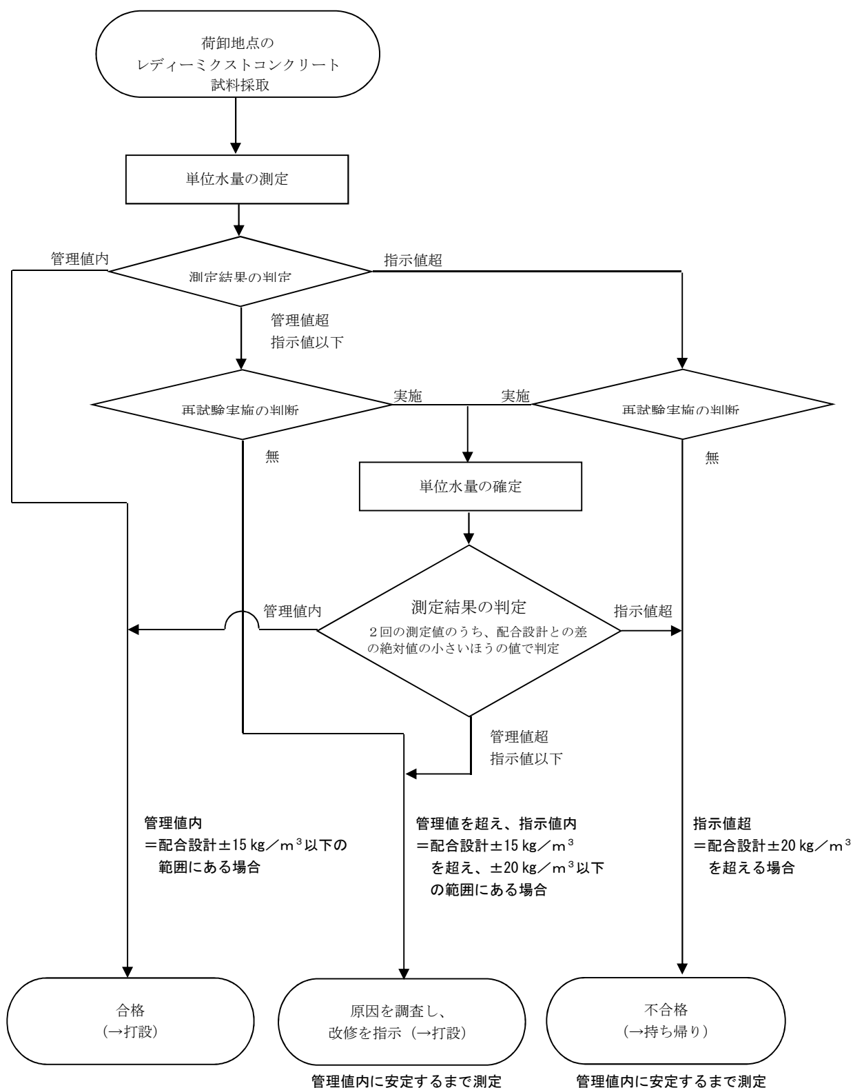
レディミクストコンクリートの単位水量測定の管理フロー図
