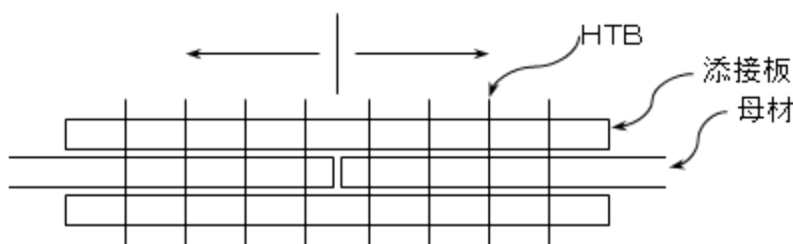
図5-1 ボルト締付け順序
