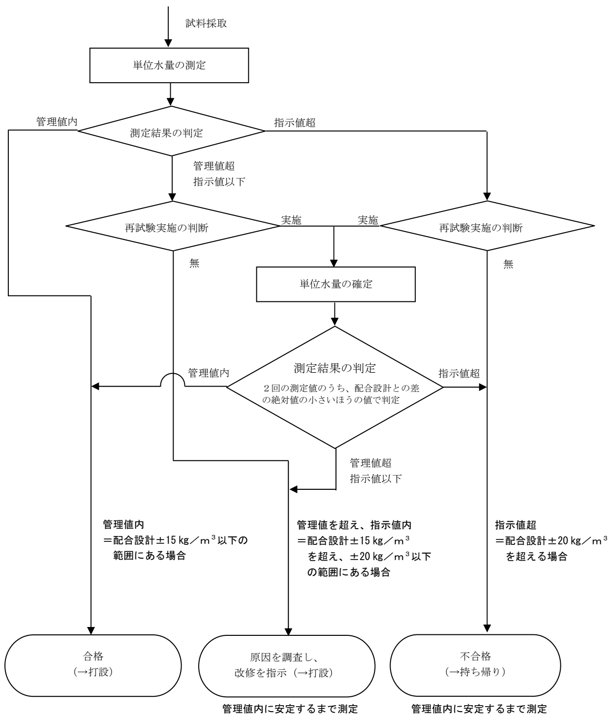
レディー-ミクストコンクリートの単位水量測定の管理フロ-図
