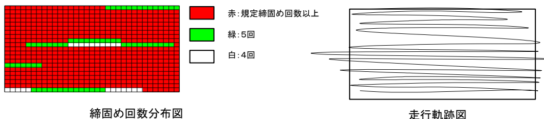
図-5 締固め回数分布図の概念図
