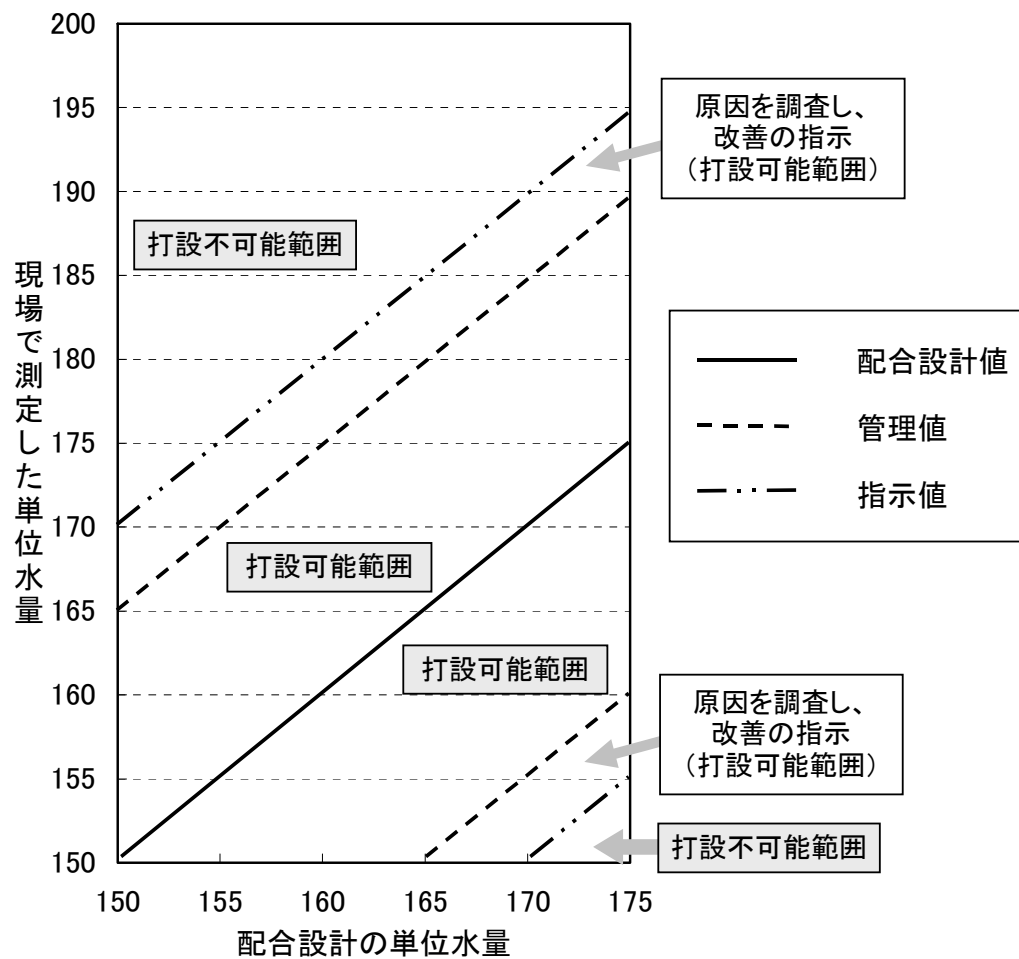
レディーミクストコンクリートの 単位水量測定の実管理図 (kg/m 3 )
