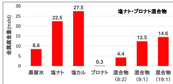
図-1 金属腐食性確認結果
