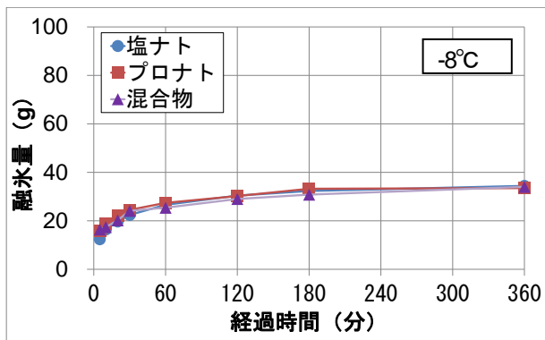
図-2 融水量の経時変化
