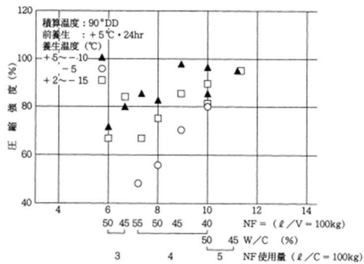
図8.2 積算温度90 D · Dにおける20℃養生の圧縮強度に対する各種養生温度の圧縮強度の比
