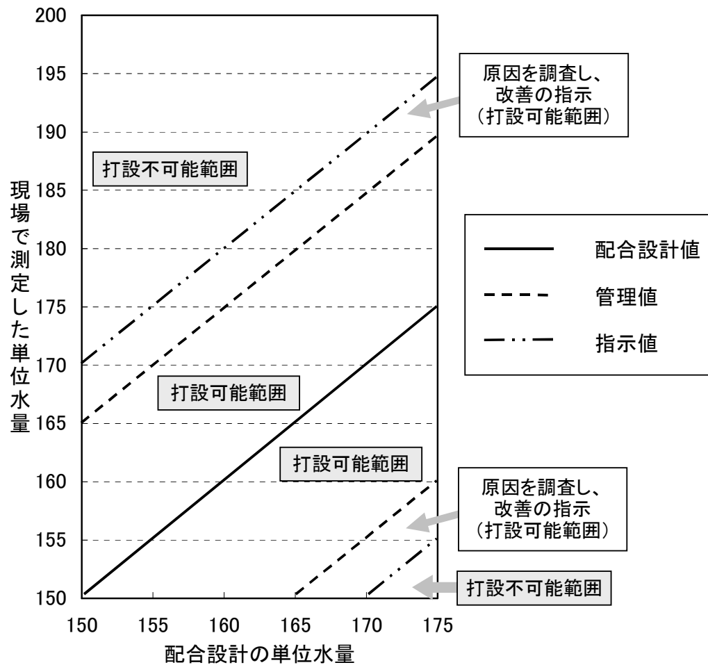
レディーミクストコンクリートの 単位水量測定の実管理図 ( \text{kg}/\text{m}^3 )
