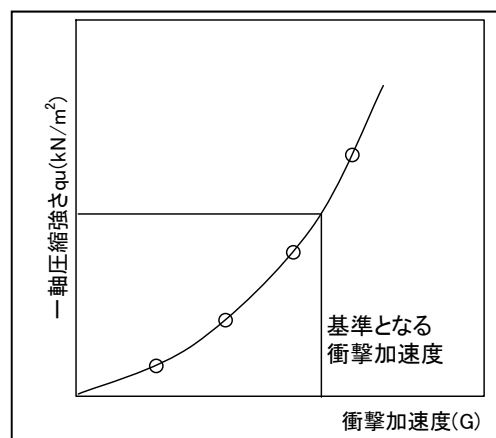
図ー５ セメントや石灰などの固化剤を改良した試料の基準となる衝撃加速度
