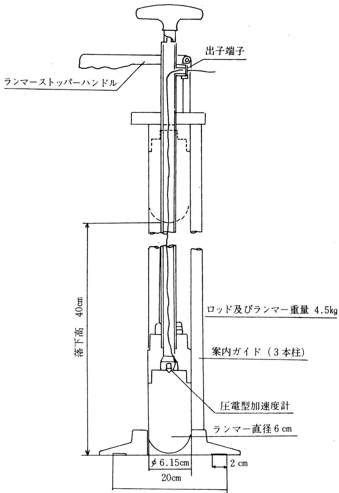
図ー 1 衝撃加速度試験器
