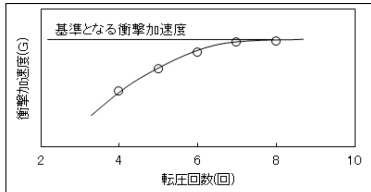
図ー４ 締め固め試験によって明確な最大乾燥密度が得られない試料の基準となる衝撃加速度
