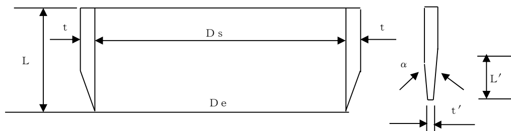
図6-1 サンプルングチューブ
