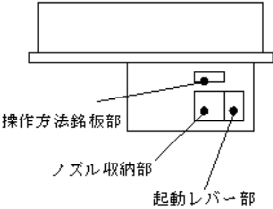
ホースリール無し式消火栓
