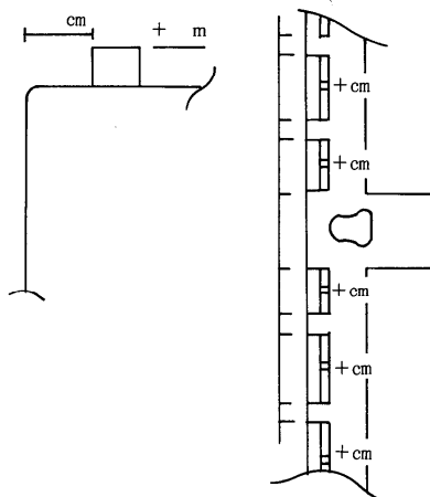
車止め出来形管理表
