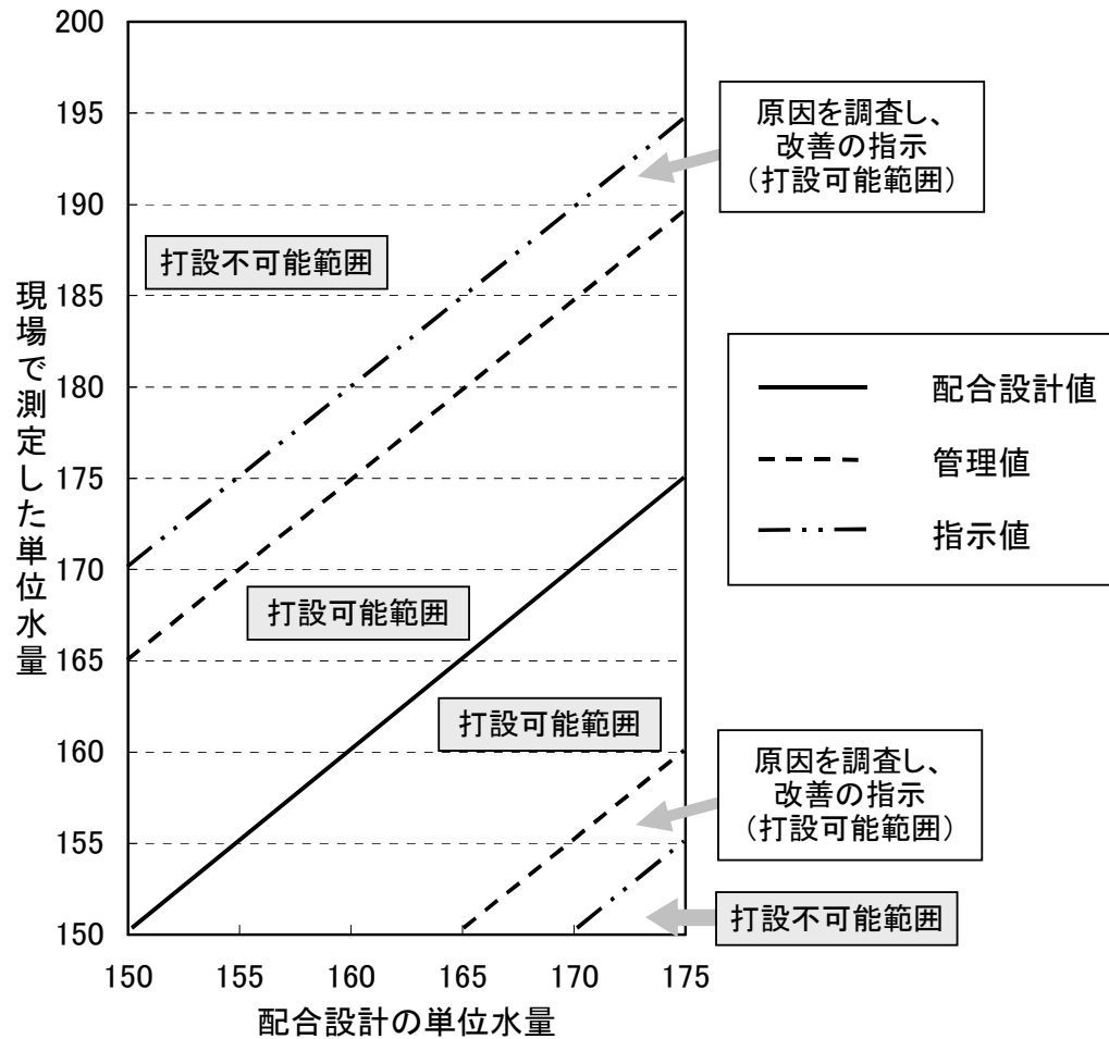
レディーミクストコンクリートの 単位水量測定管理図 ( \text{kg}/\text{m}^3 )
