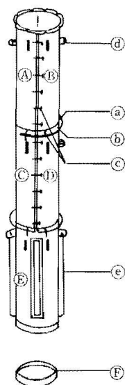
解説図 5.2.2 水中コンクリート用ケーシングの 1 例
