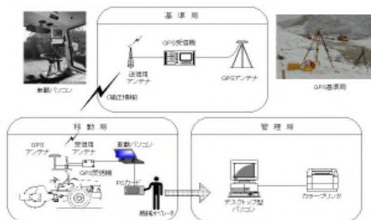
図-3 走行軌跡データの通信経路（GPS の例）
