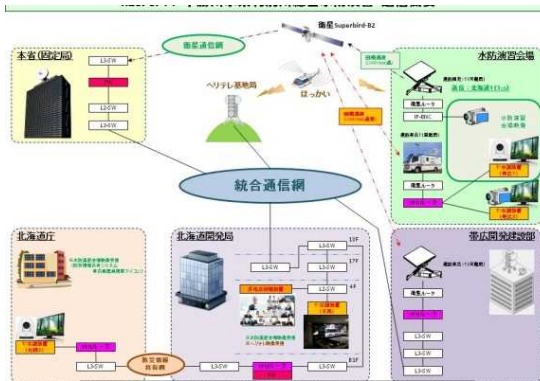
テレビ会議システム構成図
