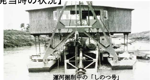
ラダーエクスカベータ掘削状況
