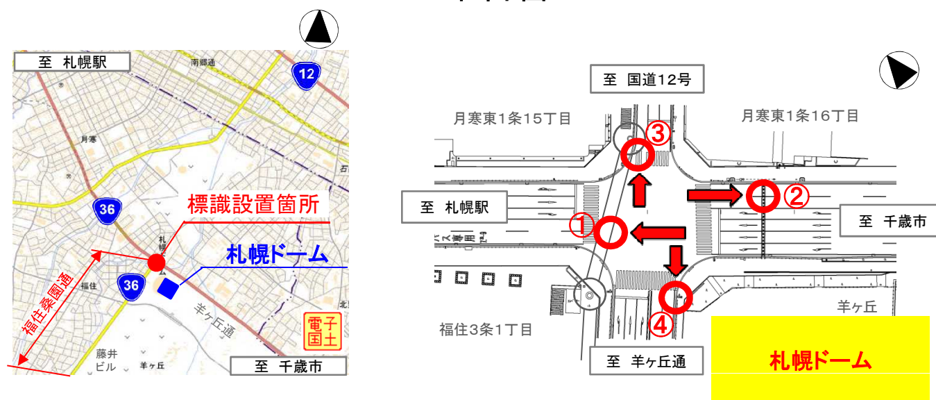
平面図
