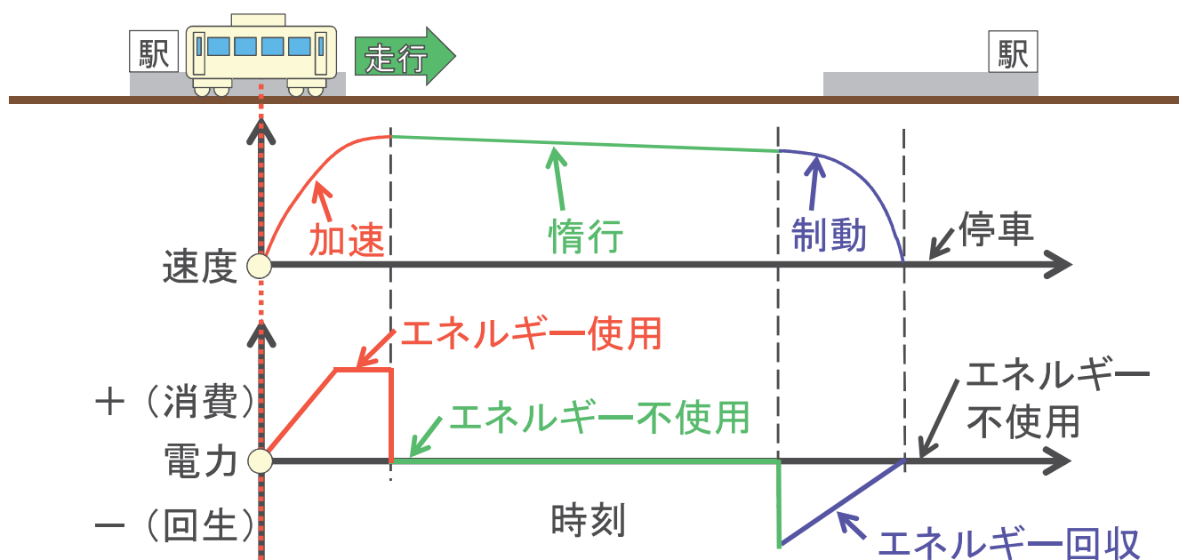
鉄道車両走行時の時刻と速度, 電力の関係
