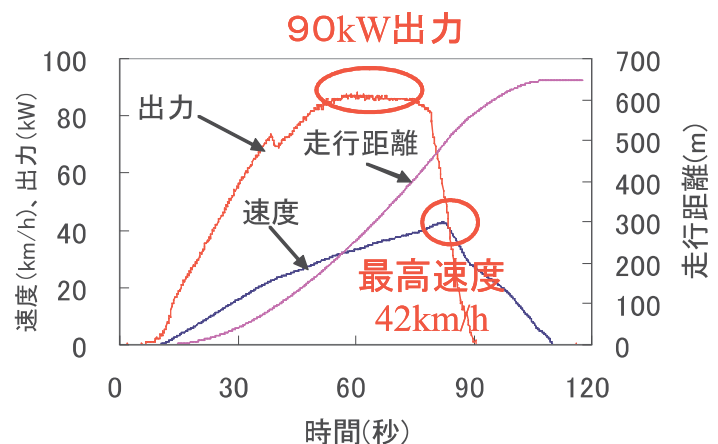
所内走行試験結果例
