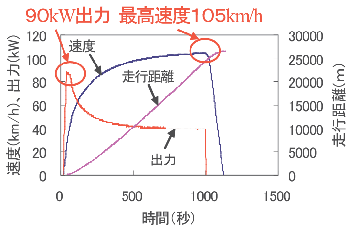
走行模擬試験結果例
