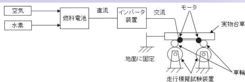
台車駆動試験構成
