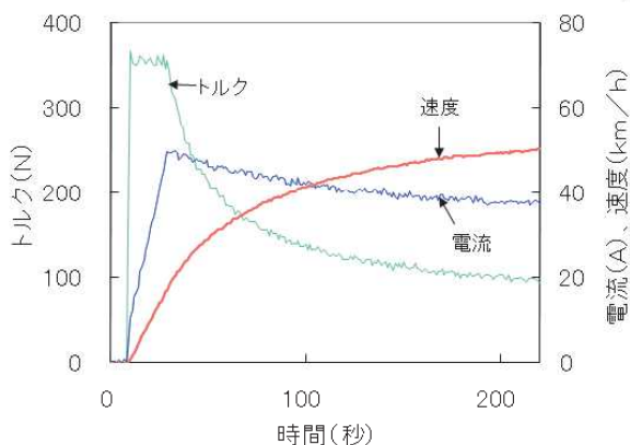
台車駆動試験結果例
