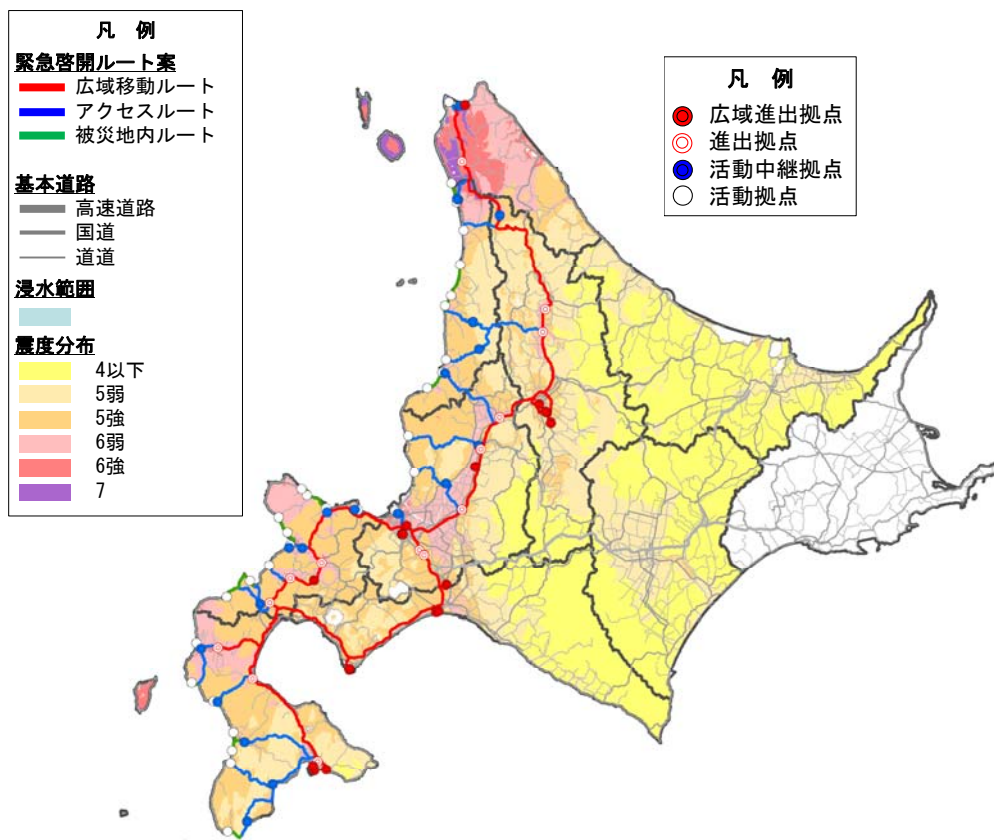
図 5 日本海地域における啓開拠点と緊急啓開ルート
