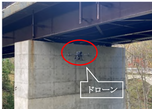
ドローンによる画像計測
