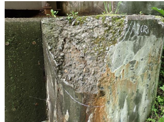
凍害による橋台の損傷
