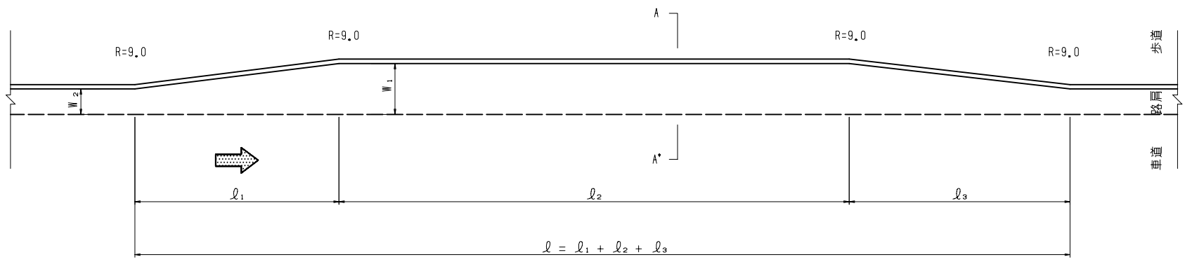
バス停車帯標準図
