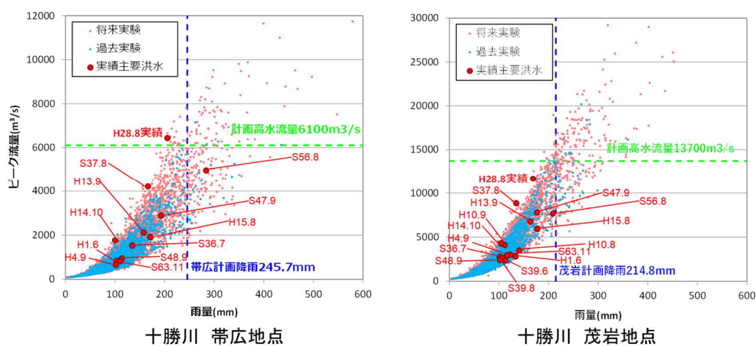
図 9 十勝川における降雨量とピーク流量の関係
