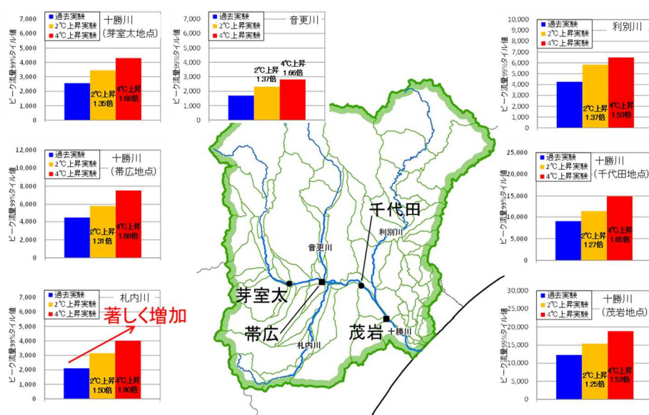
図 8 十勝川におけるピーク流量の変化倍率
