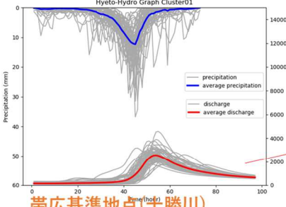
帯広基準地点(十勝川) ハイドログラフ
