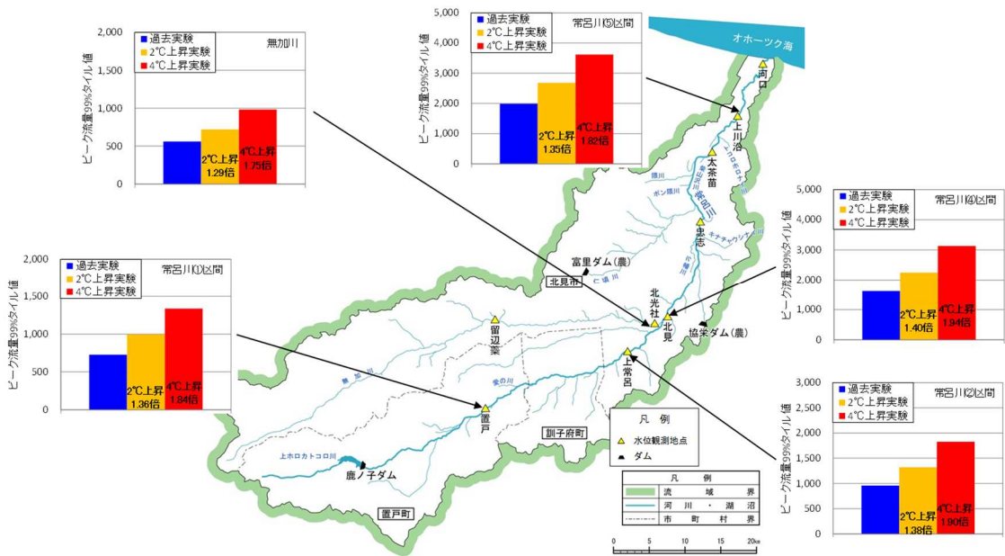
図 25 常呂川におけるピーク流量の変化倍率
