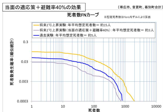
図21 当面の適応策の効果
