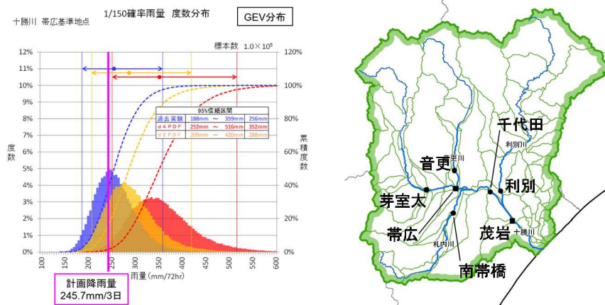
図 6 帯広地点における降雨の変化倍率
