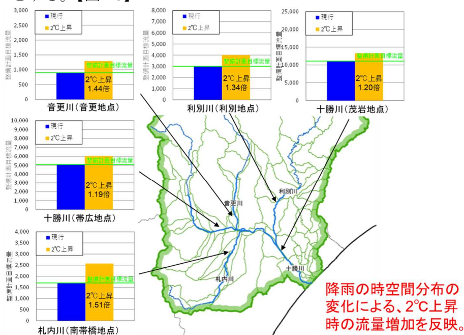
図 16 当面の治水適応策（河道掘削等）における目標流量検討例
