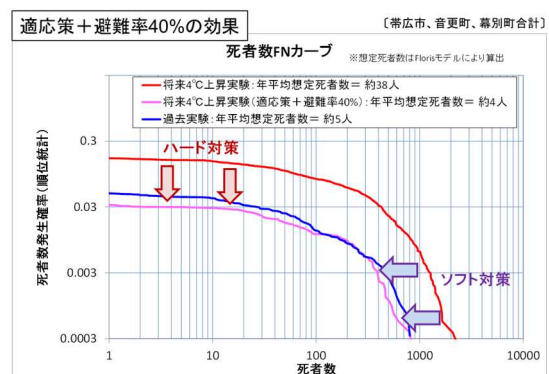
図 15 適応策の効果 (帯広市・音更町等の流域中流部の例)
