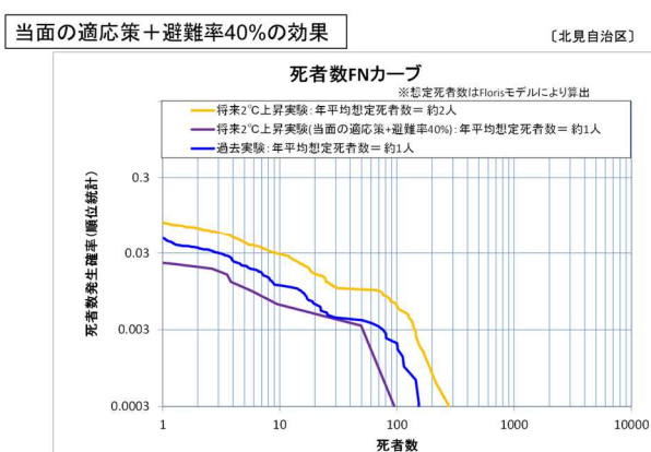
図 34 当面の適応策の効果 （北見市街地の例）
