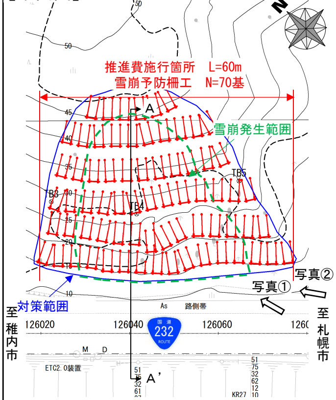
【平面図】
