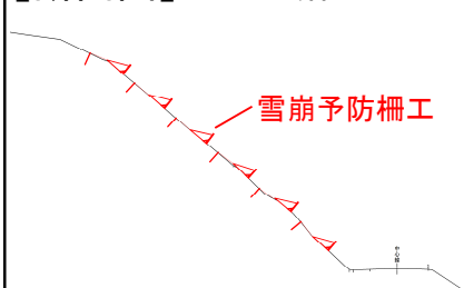
【断面図】A-A'断面
