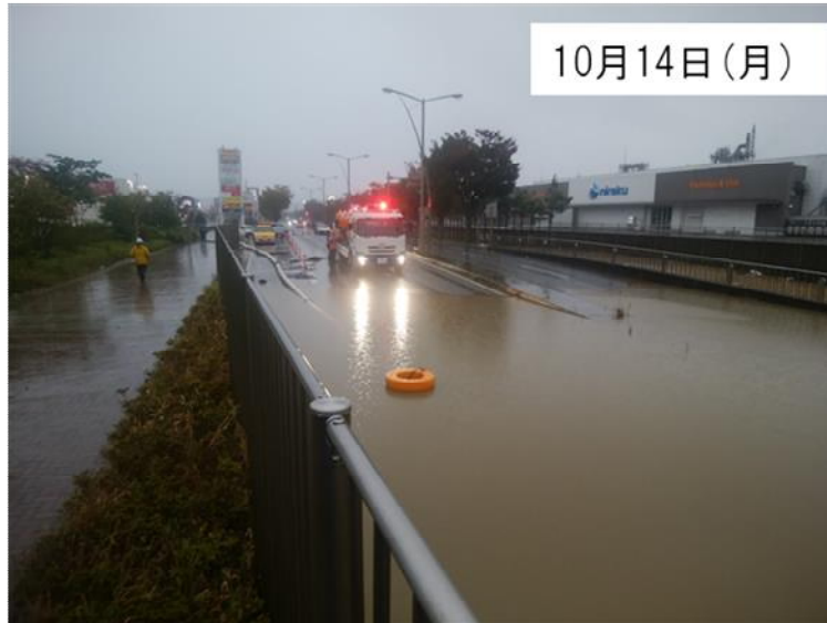
排水ポンプ車による排水作業継続中(福島県郡山市向川原町(向河原大町線アンダーパス) 応急対策班②)
