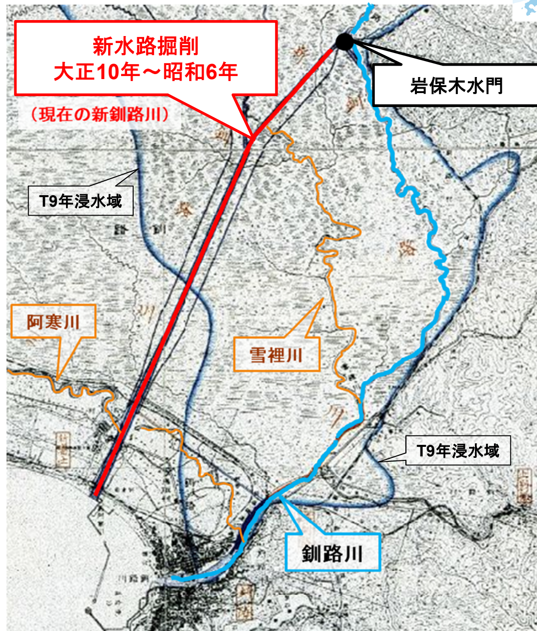
釧路川治水計画平面図(大正9年)
