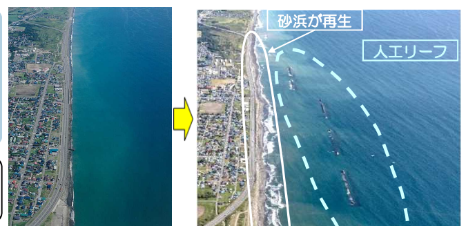
白老工区人工リーフによる砂浜の再生(左:着手前、右:整備後)
